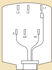
PTO3FR/PTO5FR (fused)
